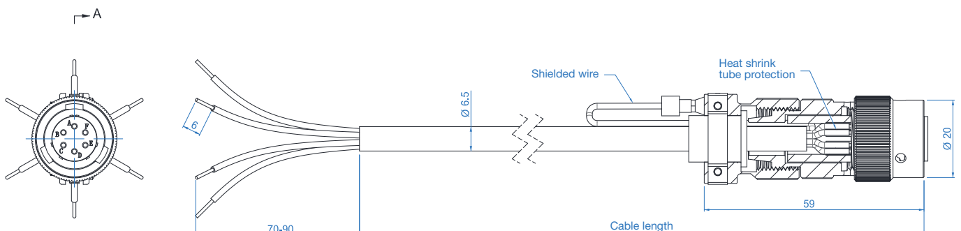
VIEW A-A
